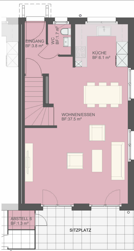
EG HAUS 6
