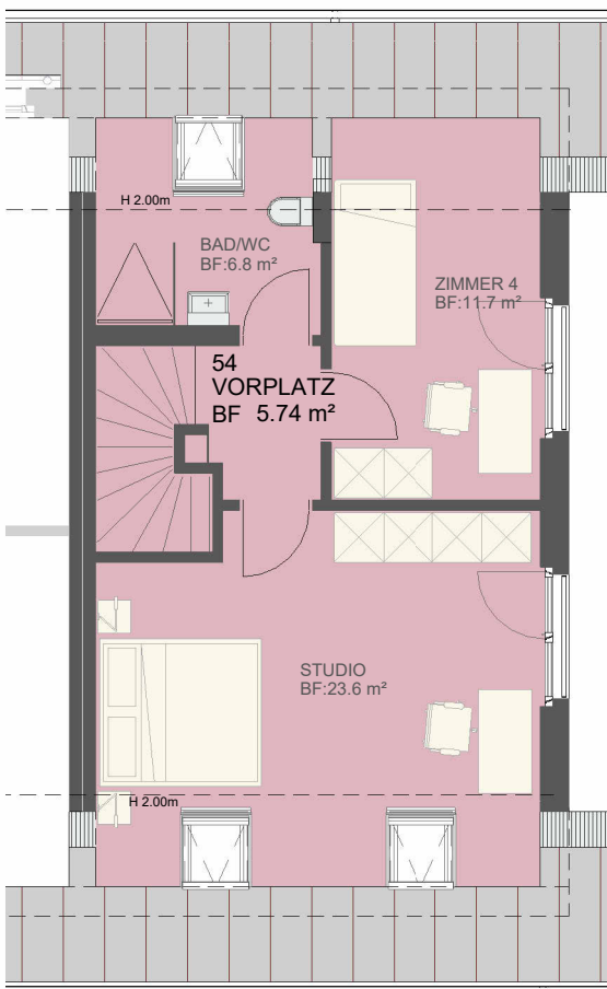
2.OG HAUS 6
