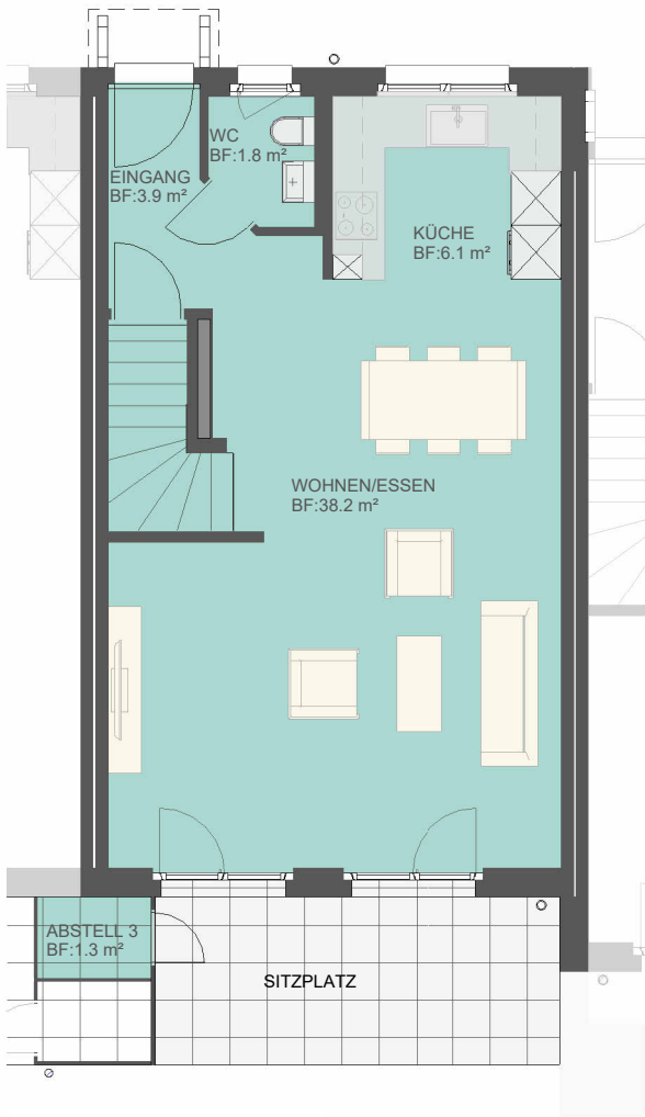
EG HAUS 3
