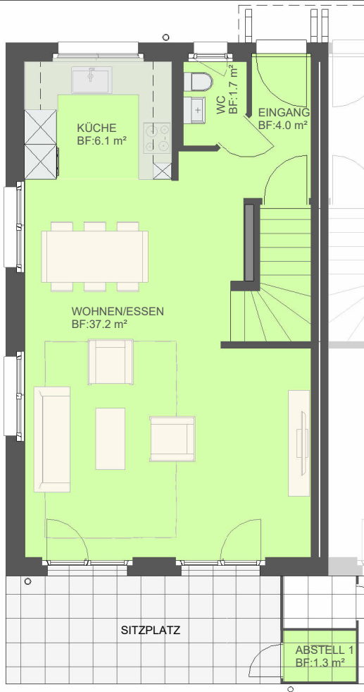
EG HAUS 1
