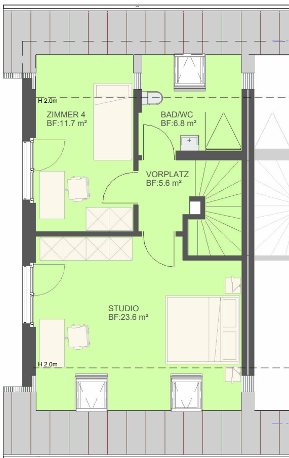
2.OG HAUS 1
