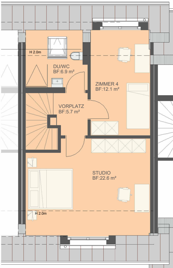
2.OG HAUS 9
