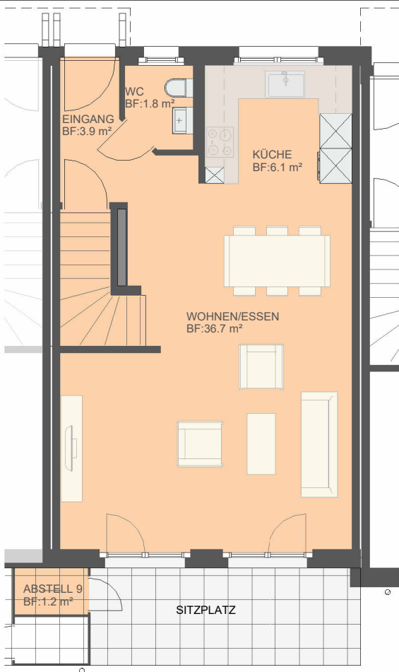
EG HAUS 9
