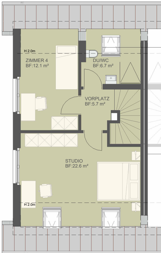
2.OG HAUS 8
