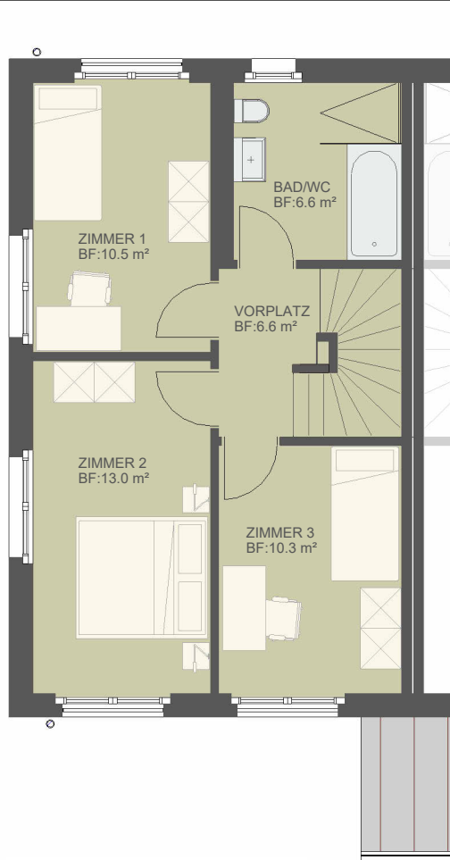
1.OG HAUS 8
