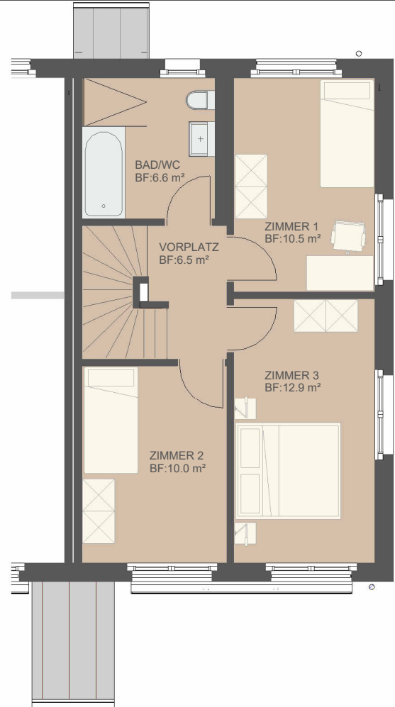
1.OG HAUS 12
