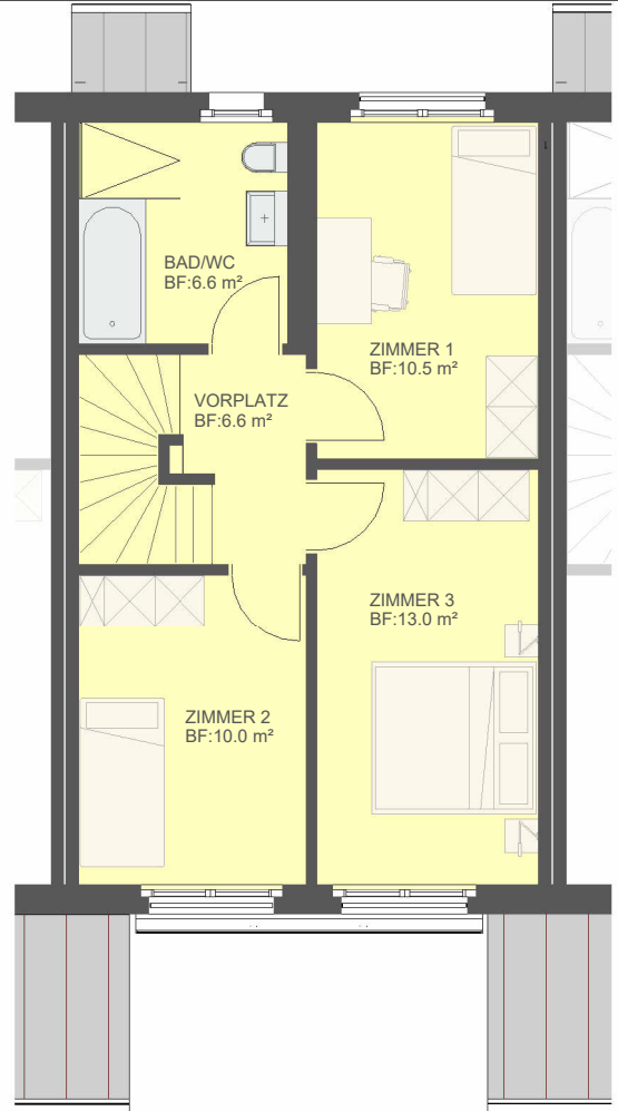
1.OG HAUS 11
