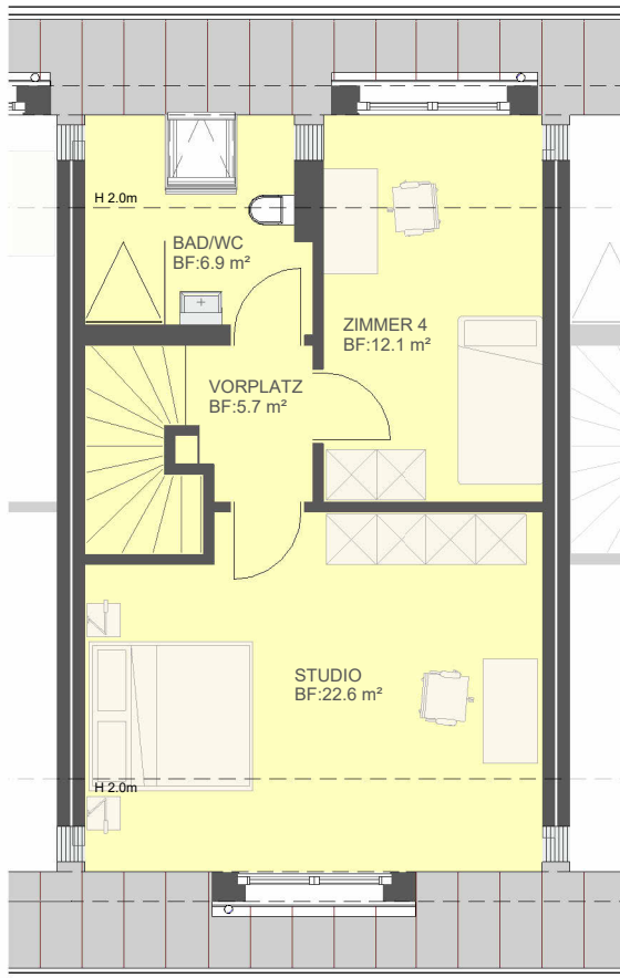
2.OG HAUS 11
