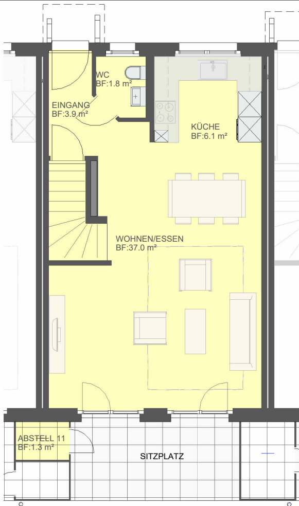
EG HAUS 11
