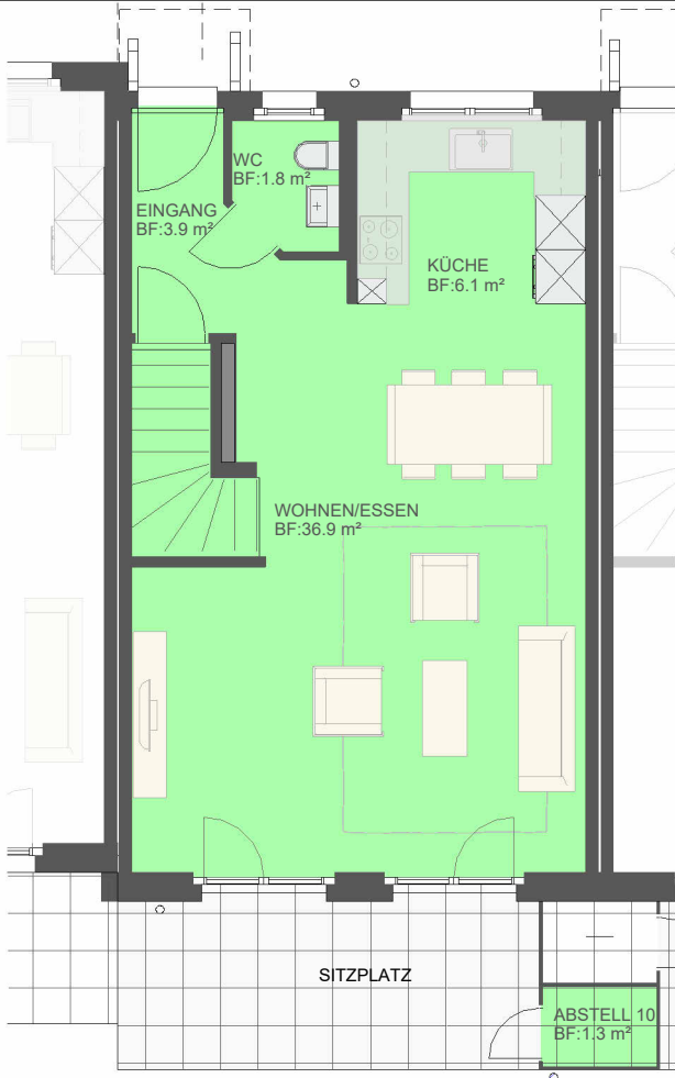
EG HAUS 10
